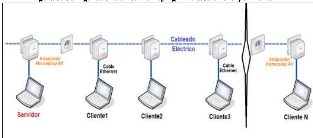
Figura 3. Configuración de Red Homeplug AV usada en el experimento
