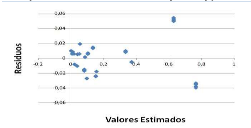
Figura 5. Valores residuales vs Valores estimados para Throughput
