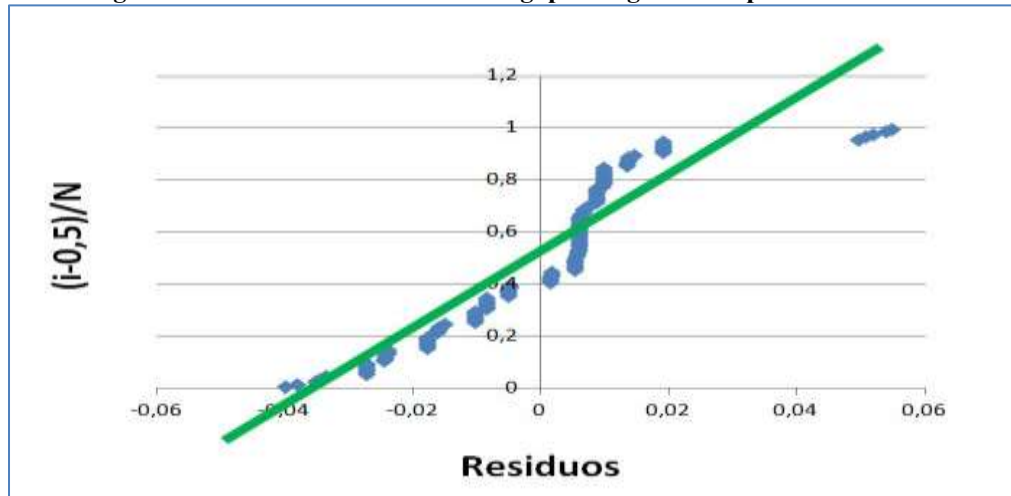
Figura 6. Valores residuales de Throughput en gráfica de probabilidad
