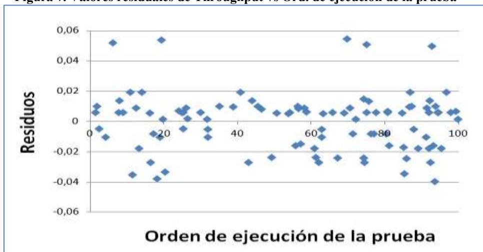
Figura 7. Valores residuales de Throughput vs Ord. de ejecución de la prueba
